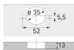
Cotes de perçage TH 52 / TH 42 Sensys, Intermat, SlideOn
