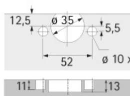
Cotes de perçage TH33 Selekta Pro 2000
