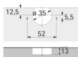
Cotes de perçage TH32 Selekta Pro 2000
