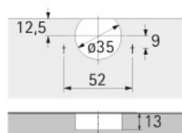
Cotes de perçage TX32/52x9 Selekta Pro 2000
