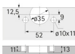
Cotes de perçage TX33/52x9 Selekta Pro 2000
