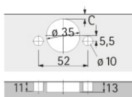
Cotes de perçage TH 53 / TH 43 / Flash / THFix Sensys, Intermat, SlideOn
