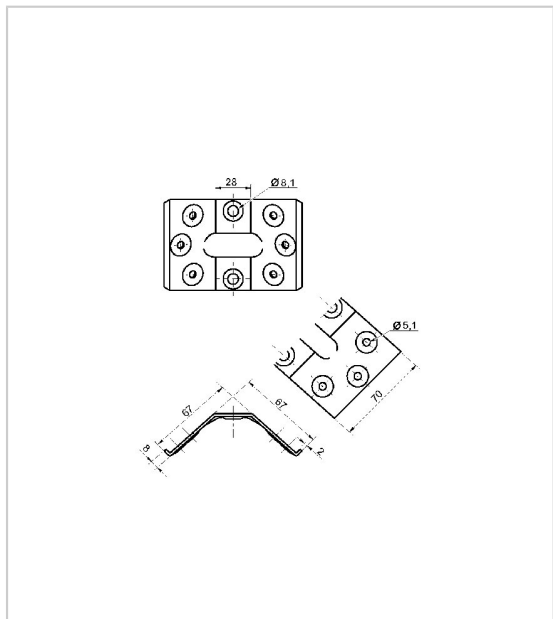
Ferrure de table acier avec retours.
