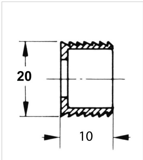
Douille d'accrochage forme trou de serrure.
